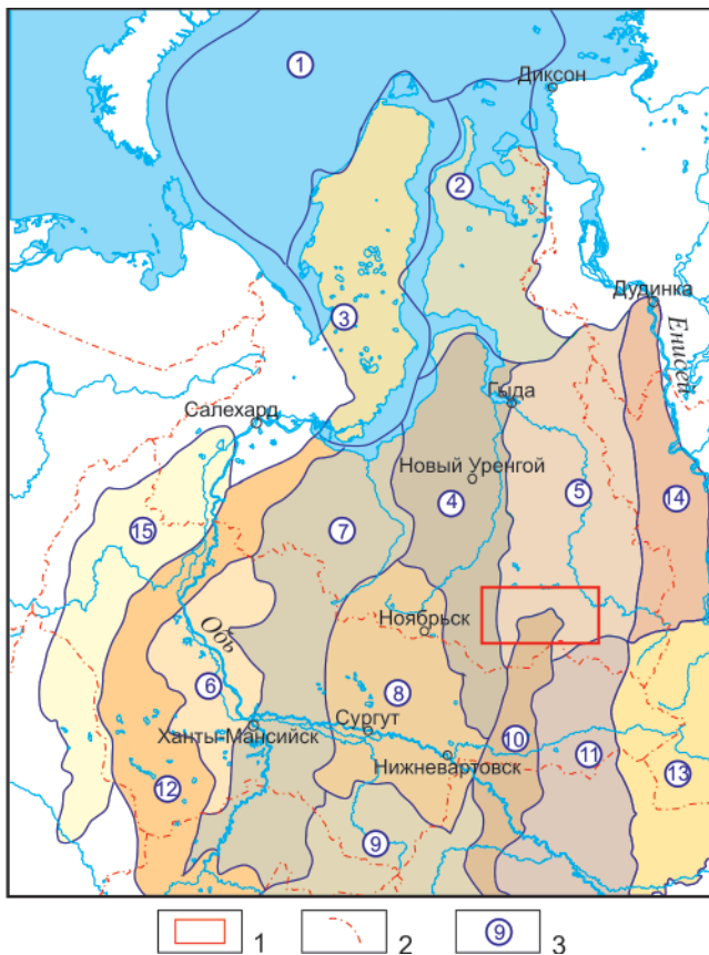
Рис. 1. Схема нефтегазогеологического районирования Западно-Сибирской нефтегазоносной провинции с указанием положения района исследования
