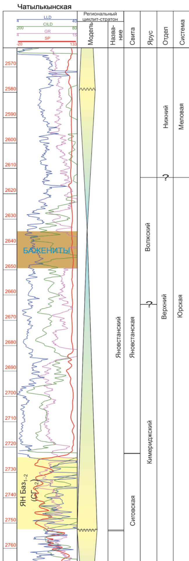
Рис. 2. Электрокаротажный образ яновстанского регионального цикллита Западной Сибири (границы ярусов и свит приведены по [9])
